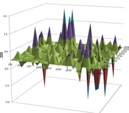
triReduceサイクル前のカウンターパーティー・リスク
