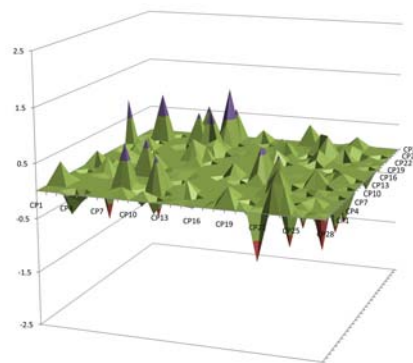
triReduceサイクル後のカウンターパーティー・リスク
